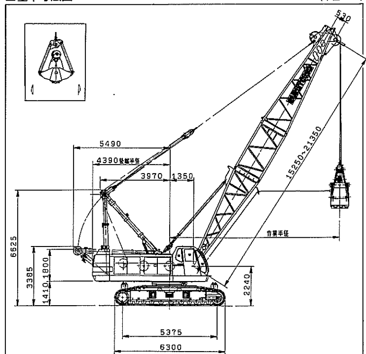
■基本寸法図
