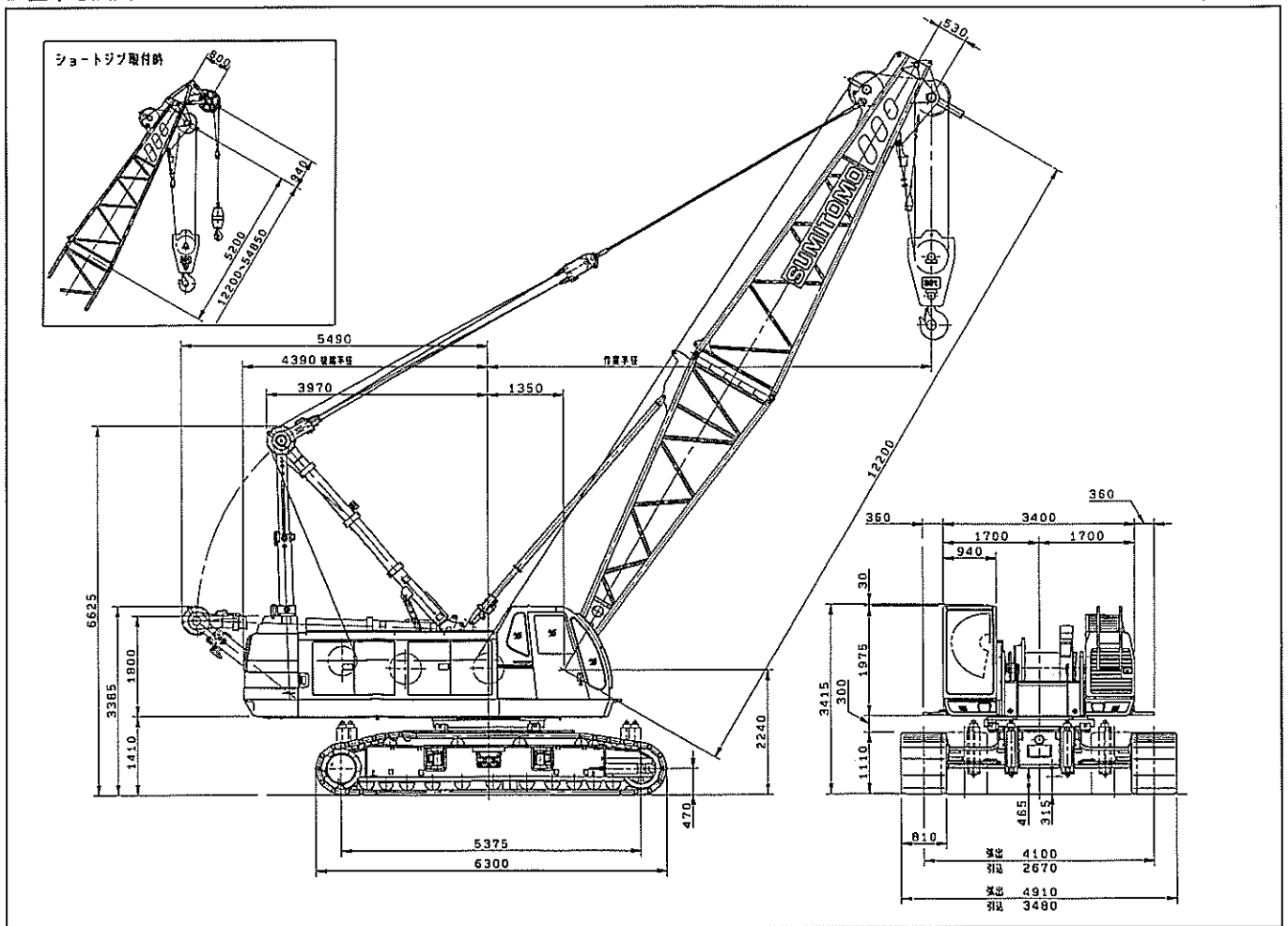
■基本寸法図
