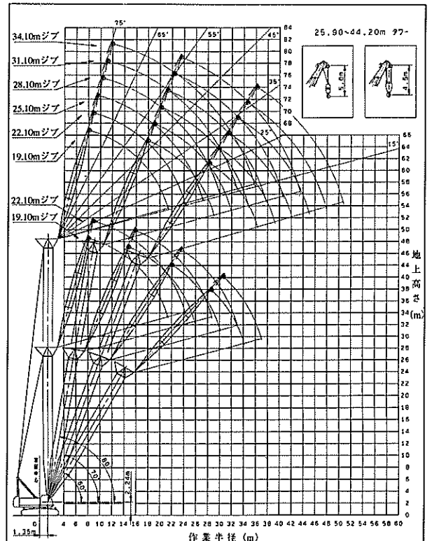
■作業範囲図
